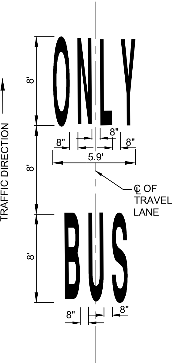
BUS ONLY WORD MESSAGE DETAIL N.T.S.
